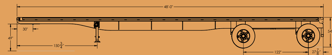
MODEL: FB-48
