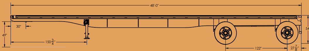
MODEL: FB-48
